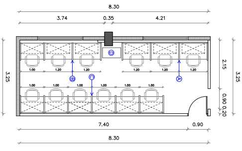
2 PLANTA AMUEBLADA DEPARTAMENTO DE AUDITORIA ESCALA 1:75
