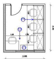
6 PLANTA AMUEBLADA OFICINA 1 DIRECCION DE LICITACIONES ESCALA 1:75
