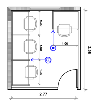
4 PLANTA AMUEBLADA OFICINA 1 DIRECCION DE LICITACIONES ESCALA 1:75
