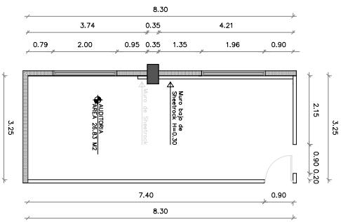
1 PLANTA DIMENSIONADA DEPARTAMENTO DE AUDITORIA ESCALA 1:75
