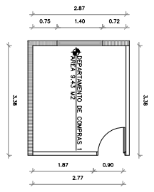
3 PLANTA DIMENSIONADA OFICINA 1 DIRECCION DE LICITACIONES ESCALA 1:75
