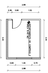
5 PLANTA DIMENSIONADA OFICINA 2 DIRECCION DE LICITACIONES ESCALA 1:75
